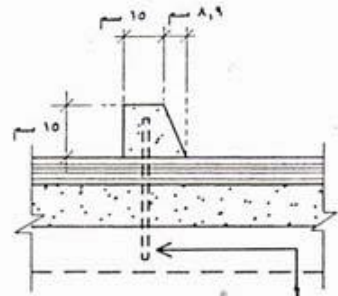
قضبان من حديد تسليح مغروسان عمودياً لتثبيت المصددة بالأرض (البعد ١٠ و ٨.٩)
